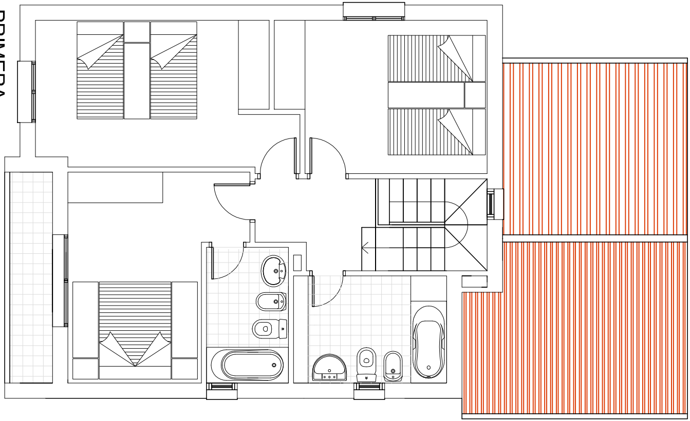
TIPO 1 (E:1/50)
